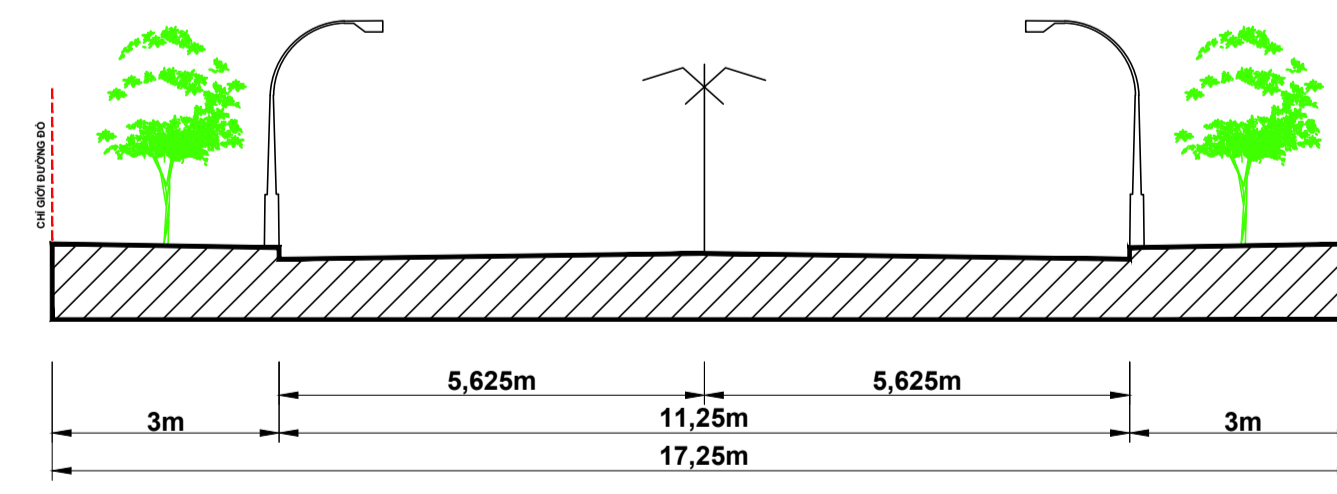
CẮT 3-3
