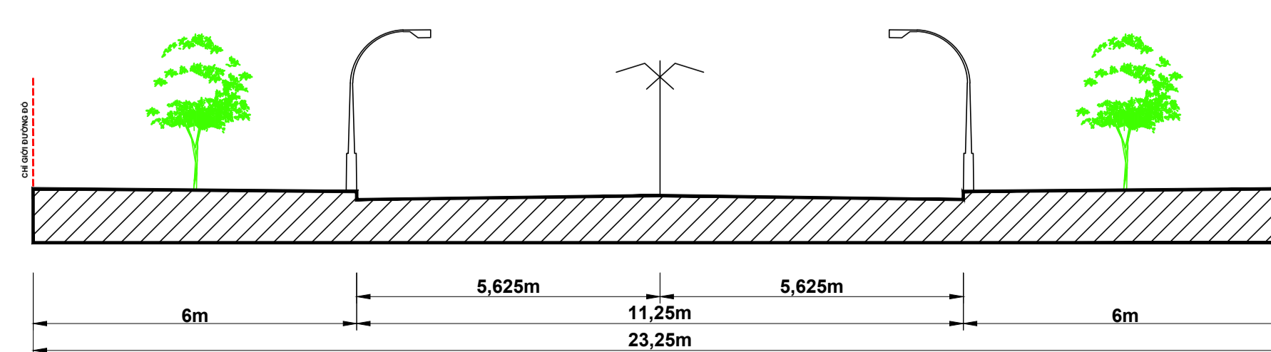
CẮT 1-1
