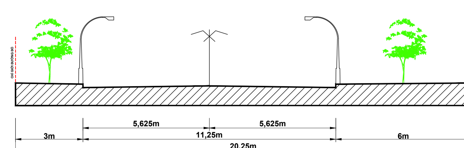
CẮT 2-2
