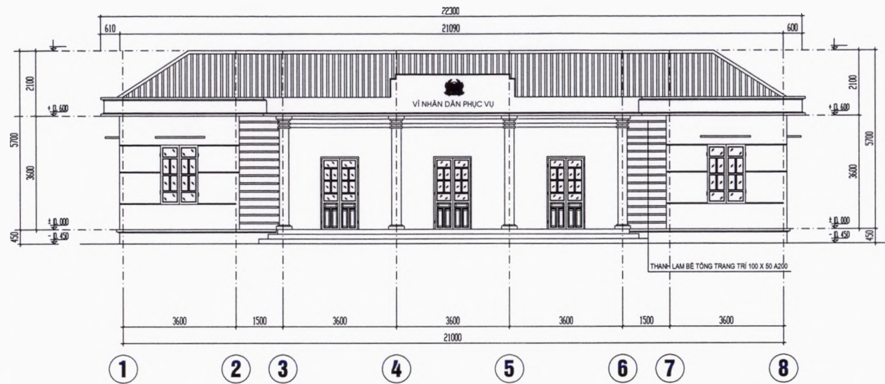
MẶT ĐỨNG TRỰC 1 - 6
