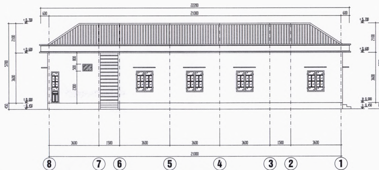
MẶT ĐỨNG TRỰC 8 - 1
