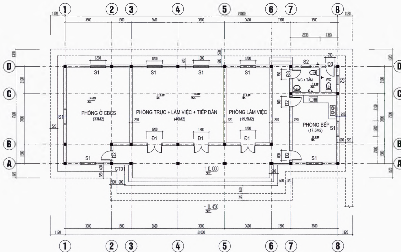
MẶT BẰNG COS +0.000
