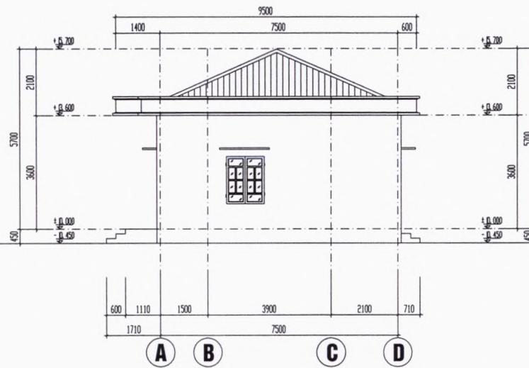
MẶT ĐỨNG TRỤC A - D
