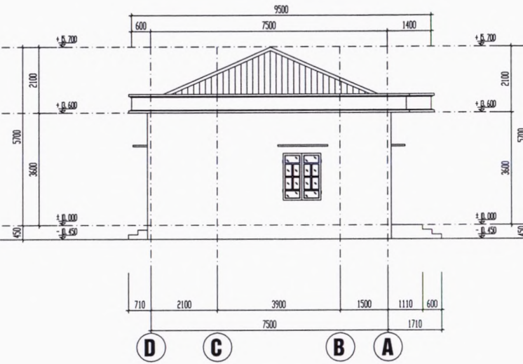
MẶT ĐỨNG TRỤC D - A
